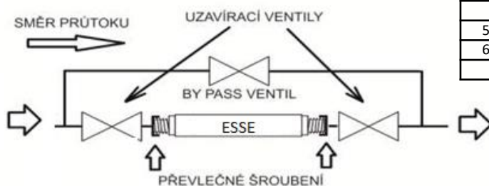
Schéma zapojení
