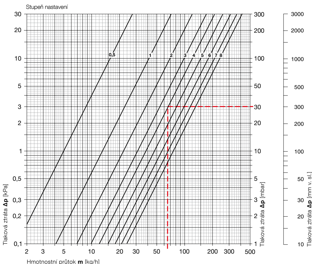
Ventil s termostatickou hlavíčí
